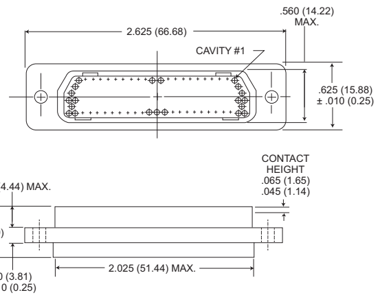
Receptacle
