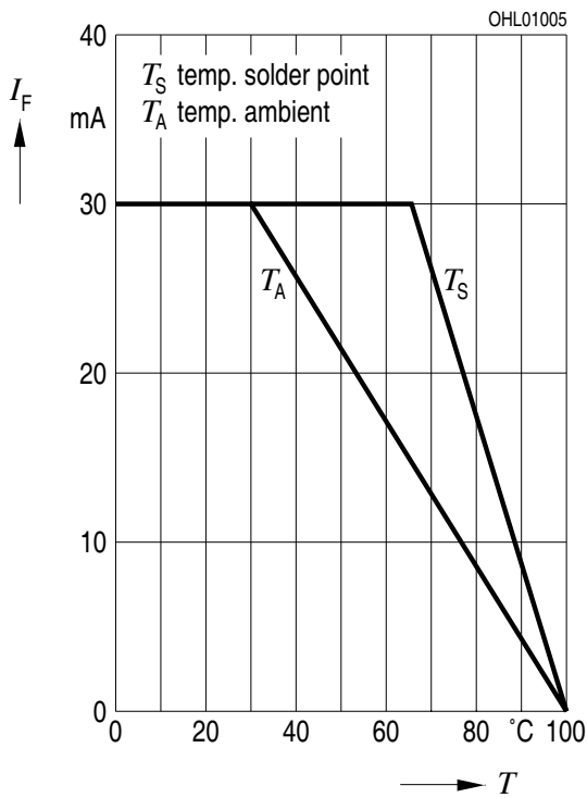
Maximal zulässiger Durchlaßstrom I_F = f(T) Max. Permissible Forward Current
